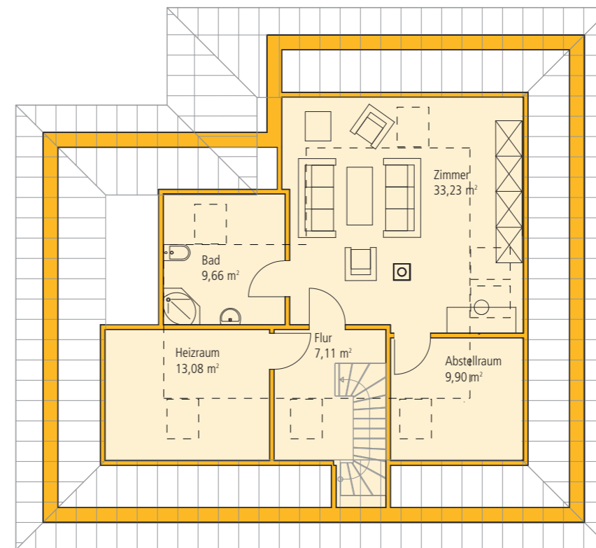
Dachgeschoss
